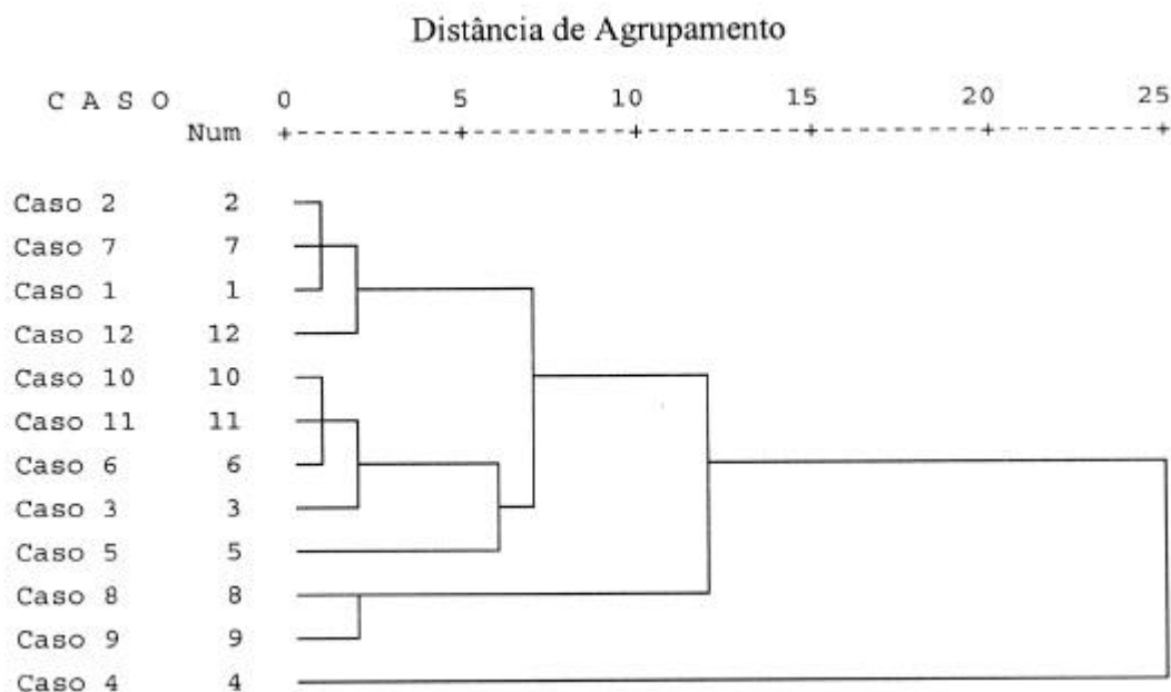
Dendrograma 1 - Análise de cluster usando Average Linkage (Between Groups) para o ano de 1991
