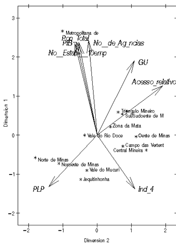
Gráfico 3 – ACP para o ano de 2000
